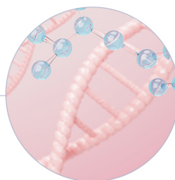
Biceridový complex
